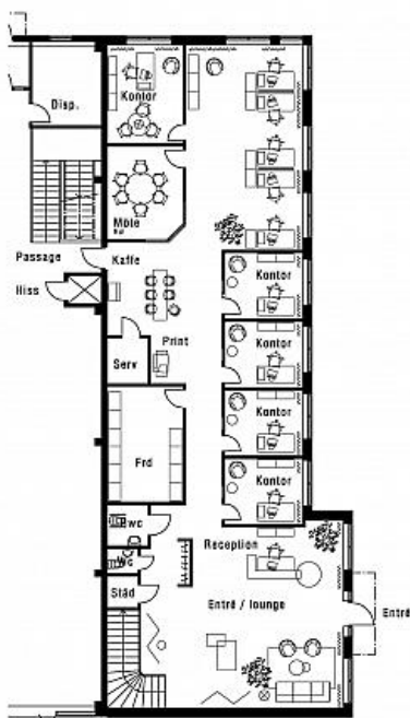
Plan 1 - Möbleringsplan
